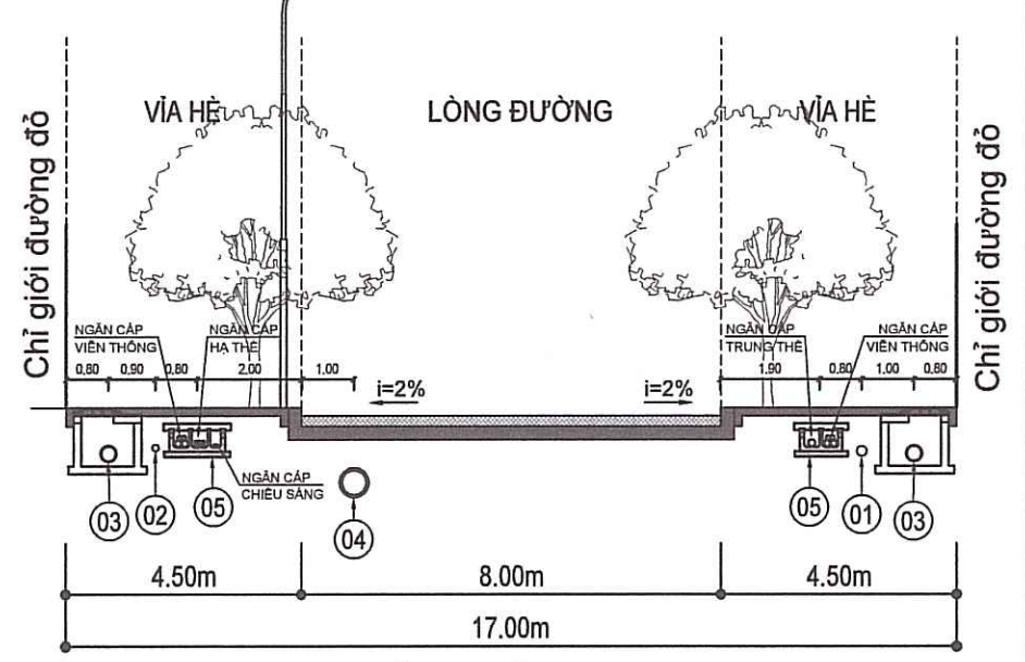
MẶT CẮT 1-1
