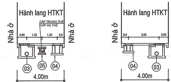
MẶT CẮT 3-3 MẶT CẮT 4-4
