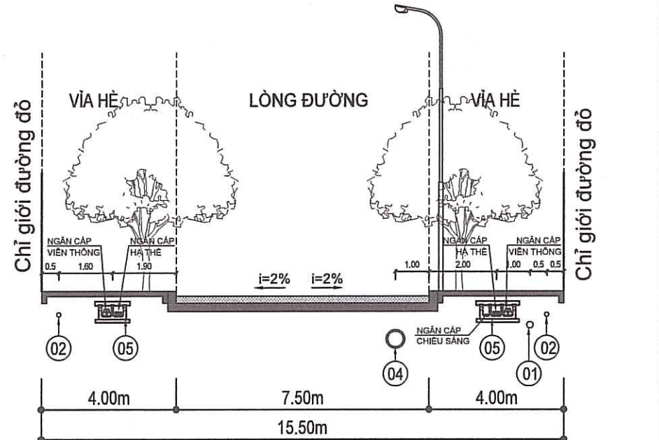
MẶT CẮT 2-2
