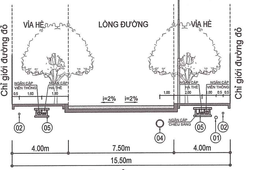
MẶT CẮT 2-2
