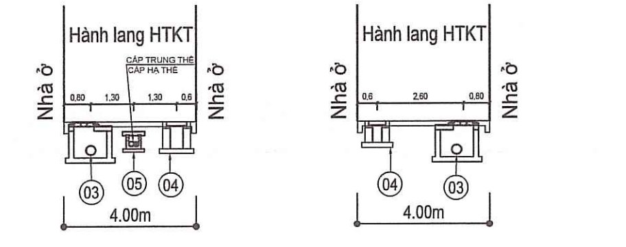
MẶT CẮT 3-3 MẶT CẮT 4-4
