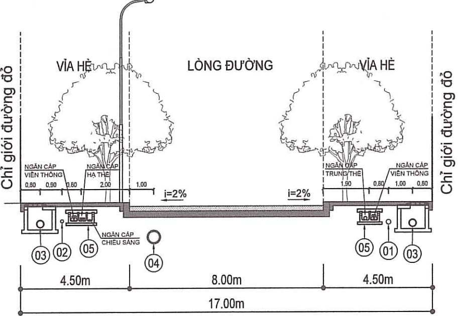
MẶT CẮT 1-1
